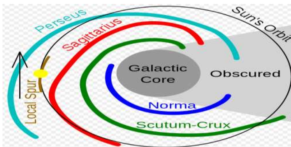
Fig. I.1 - Estrutura da Via Láctea - Neste esquema, o Braço de Órion é rotulado "Local Spur". A posição do Sistema Solar é indicado pelo “ponto amarelo” – Fonte: Wikipedia.
